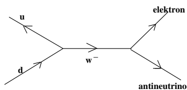
14. ábra. Neutron protonná való bomlásakor a neutron belsejében egy d kvark u kvarkká alakul. Eközben egy hipp-hopp W^- bozon keletkezik, ami elektronná és ellenneutrínóvá (antineutrínóvá) bomlik el.
